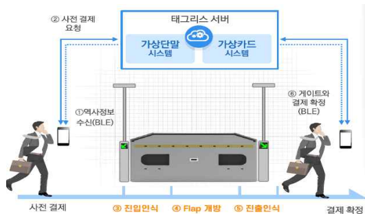
< 비접촉(태그리스) 결제 흐름도 >
