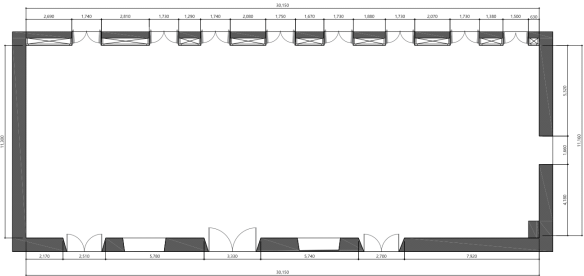
<기획전시실 도면, 340㎡>
